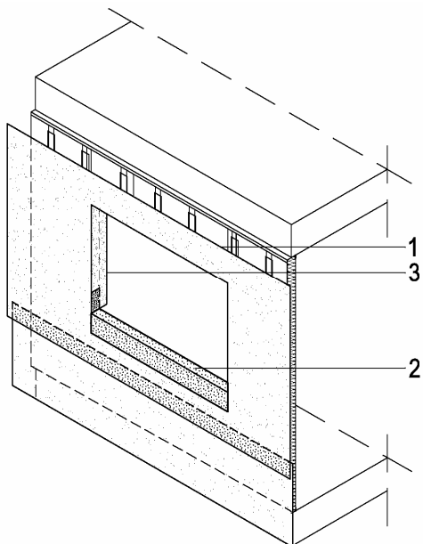
Figura 6.19.b: Vista 2 del montaje de la lámina.
