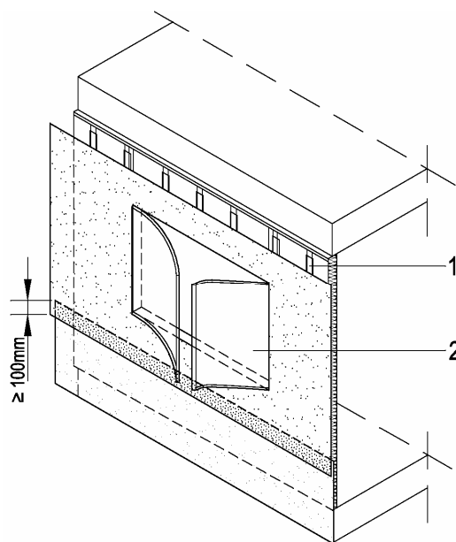
Figura 6.19.a: Vista 1 del montaje de la lámina.
