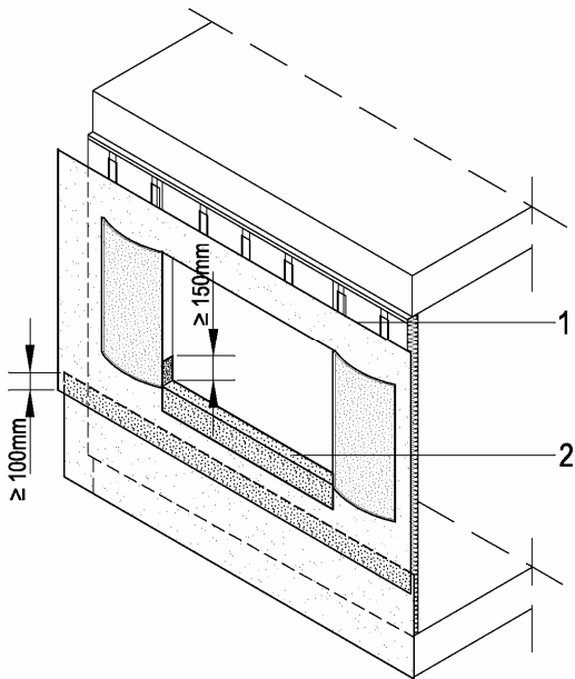
Figura 6.19.b: Vista 2 del montaje de la lámina.
