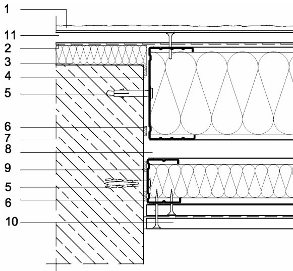
Figura 6.2: Sección horizontal del sistema Aquapanel® Outdoor W388 (W387).
