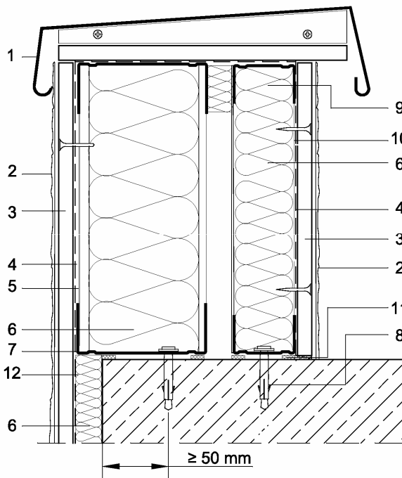
Figura 6.9: Encuentro con jamba y persiana W388 (W387).
