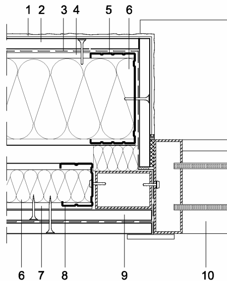
Figura 6.8: Encuentro con jamba W388 (W387).
