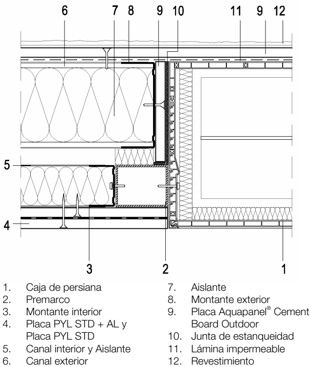
Figura 6.9: Encuentro con jamba y persiana W388 (W387).
