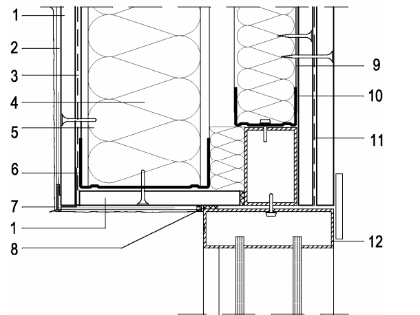
Figura 6.11: Encuentro con forjado W388 (W387).
