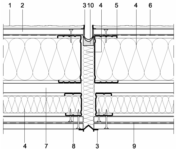
Figura 6.4: Junta de control superficial del sistema Aquapanel® Outdoor W388 (W387).
